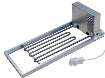
Nachheizungskassette
